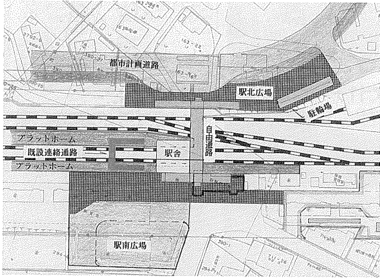
当別駅周辺の整備計画概要図
