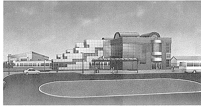
▲自由通路・当別駅舎の橋上化 当別駅舎や線路で分断されている町の南北とを結ぶ「自由通路」建設（委託）と、狭小で老朽化が進む当別駅舎を改築（JR北海道へ費用負担）します。自由通路、駅舎は鉄骨造2階建て、総建築面積約1,400平方メートルで、1階は階段や2基のエレベーター、1カ所のトイレ。2階は待合室や駅事務所で、平成6年度に完成します。
